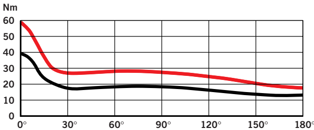
Momentkurve DORMA TS 93 (Lukkekräftinnstilling EN 5) — Åpningsmoment — Lukkemoment
